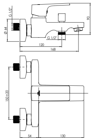
MODENA-10 Wall bath faucet MD10008 | MD10L08 (Lux)*
