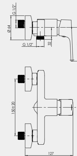
MODENA-12 Shower faucet MD20008 | MD20L08 (Lux)*
